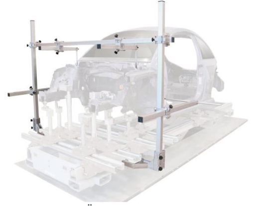
McPherson Ön düzen üst ölçüm Sistemi
